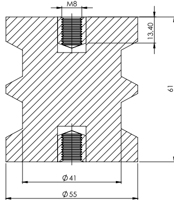
Mesnet İzolatör (M8) / Insulator (M8)
